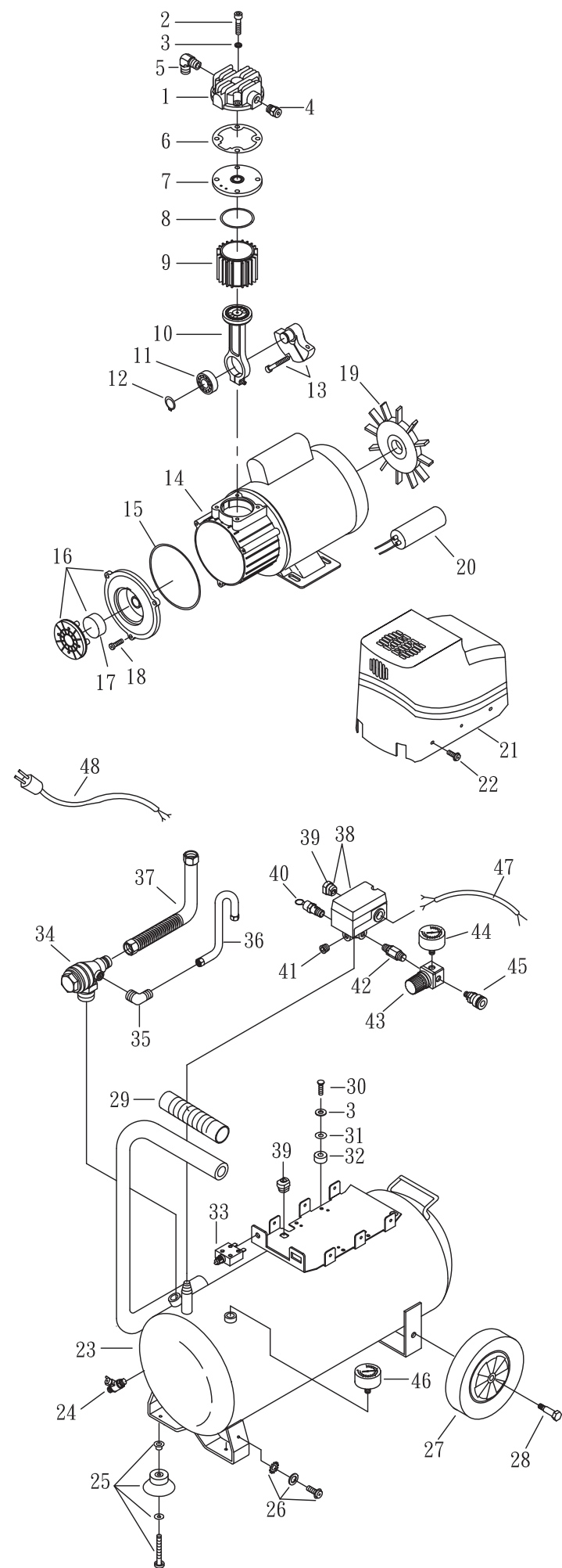
SR-102 分解図
